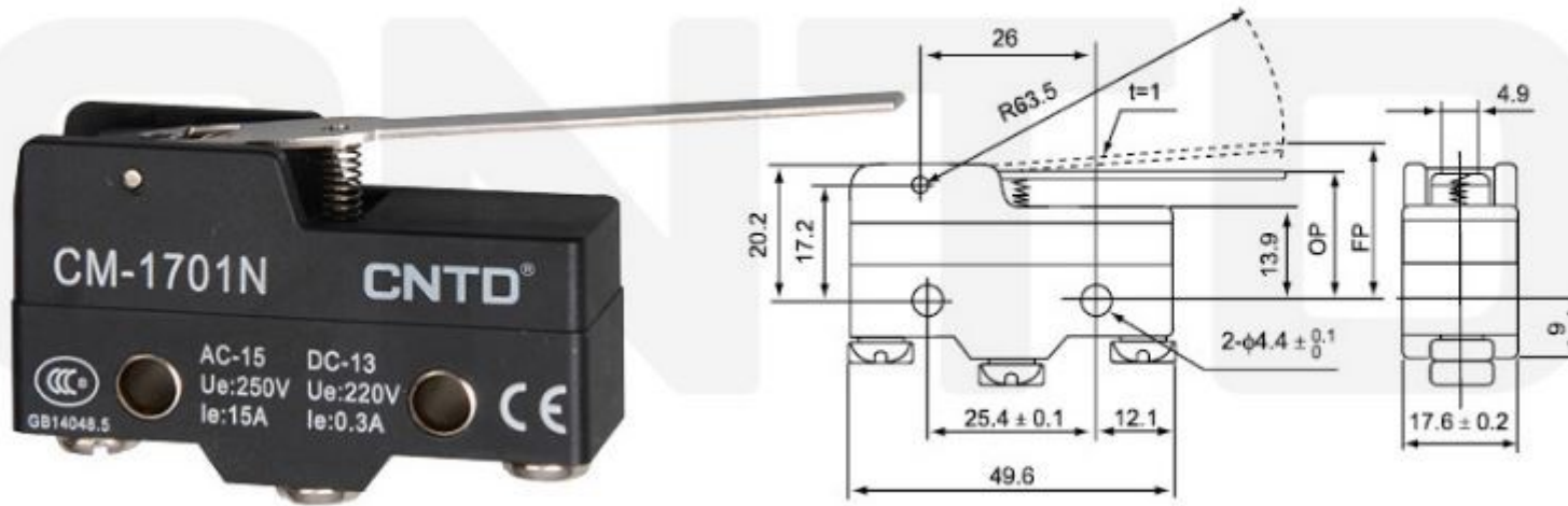
CM-1701N
